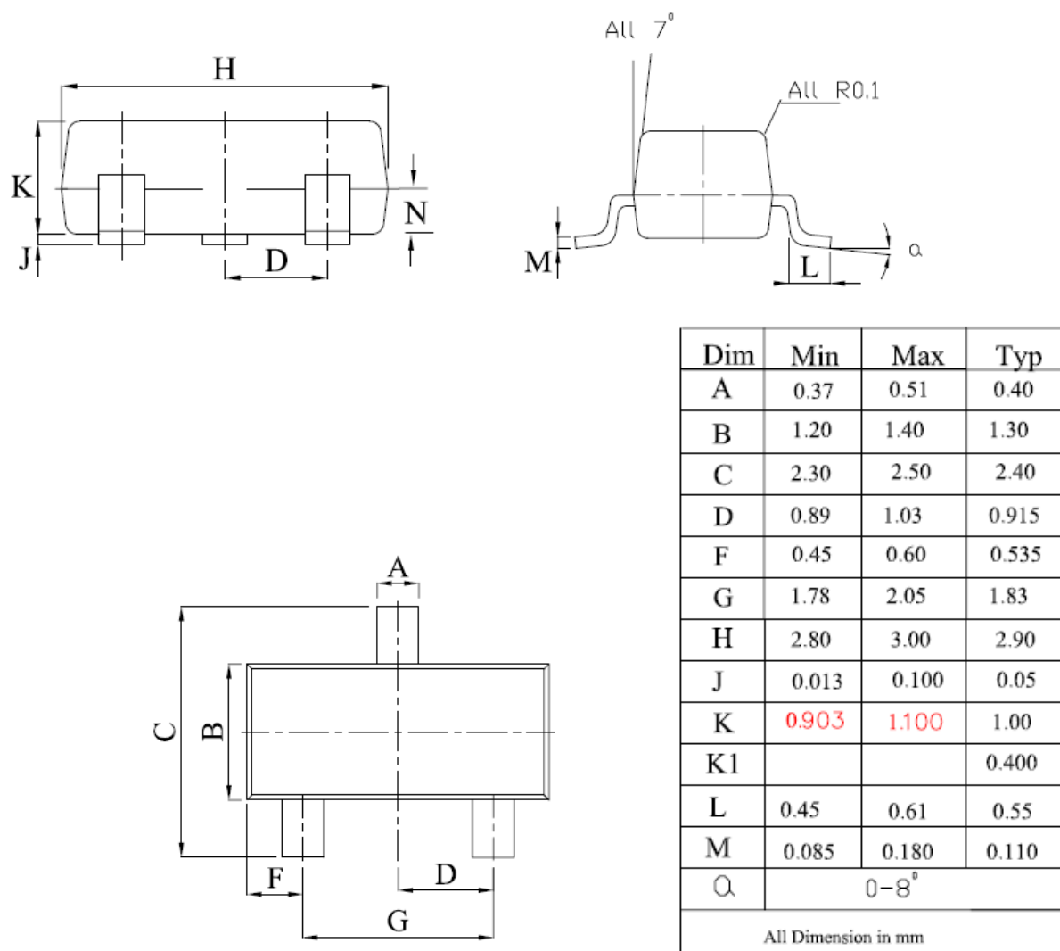
图 4. S0T23-3 封装尺寸
